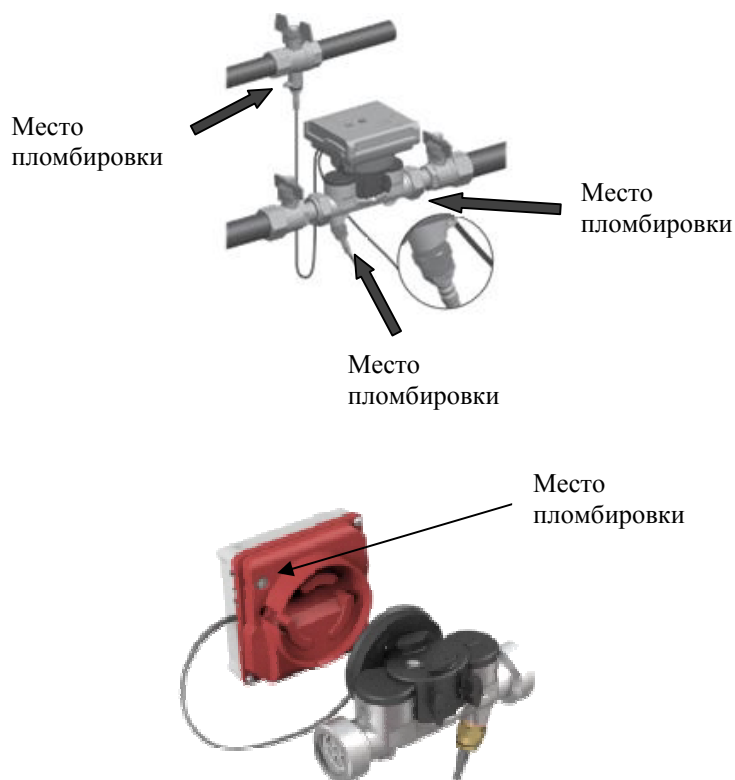
Рис. 5 - Места пломбировки теплосчетчиков CF, модели CF-UltraMaXX V, CF-UltraMaXX МК
